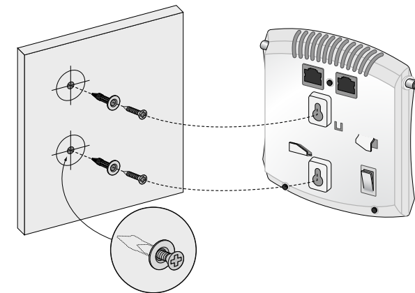
图 4 在墙壁上安装 W-AP90 系列接入点
