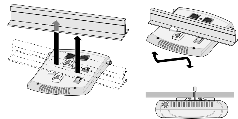
图 5 调整吊顶板轨道安装槽的方向
