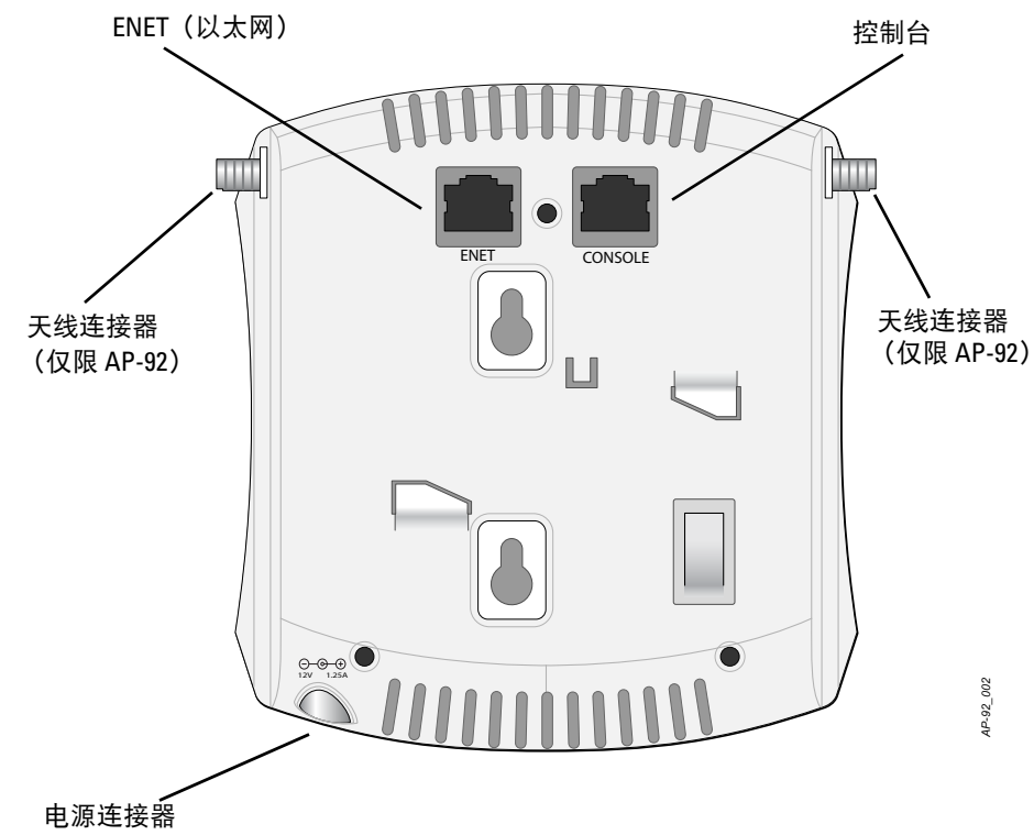
图 3 后部（所示为 W-AP92）
